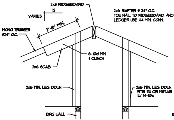
CONV. FRAMING DETAIL SCALE: N.T.S.
