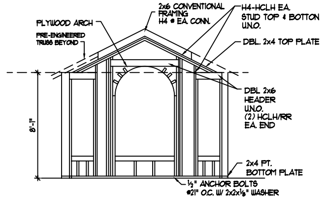
BAY ELEVATION SCALE: N.T.S. 6-8-91
