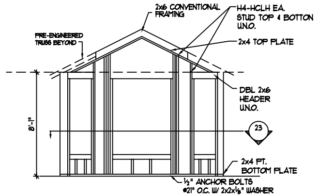
BAY ELEVATION SCALE: N.T.S. F 6-8-91
